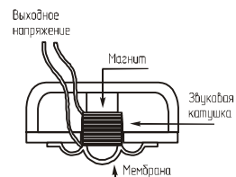
Внутреннее устройство динамического микрофона
