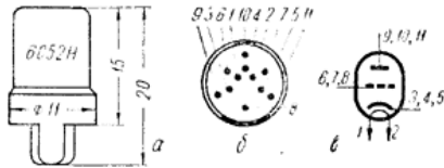
Рис. 516. Лампа 6С52Н: а — основные размеры; б — вид со стороны выводов; в — схематическое изображение; 1 и 2 — подогреватель (накал); 3, 4 и 5 — катод; 6, 7 и 8 — сетка; 9, 10 и 11 — анод.
