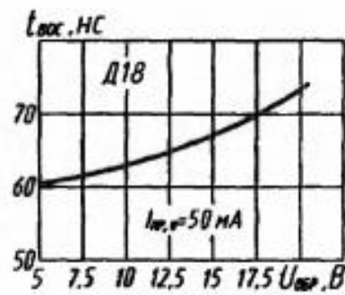
Зависимость времени обратного восстановления от обратного напряжения
