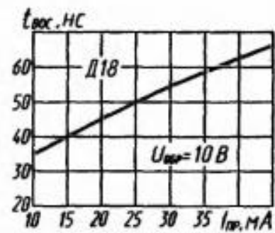
Зависимость времени обратного восстановления от прямого тока
