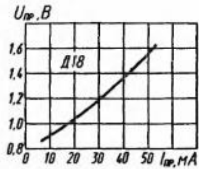
Зависимость прямого напряжения от прямого тока
