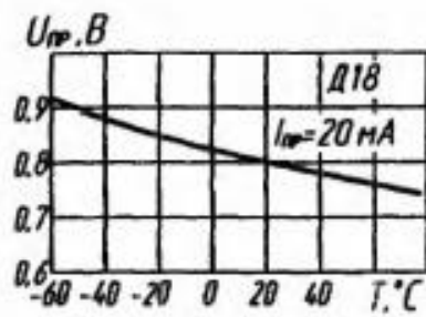
Зависимость прямого напряжения от температуры
