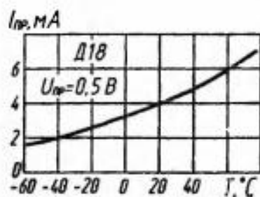
Зависимость прямого тока от температуры
