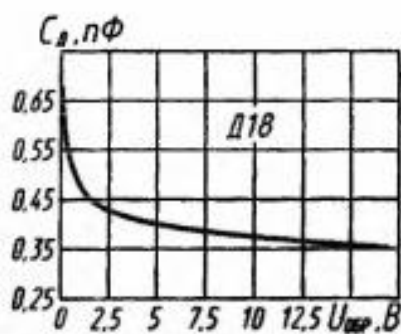
Зависимость общей емкости диода от напряжения
