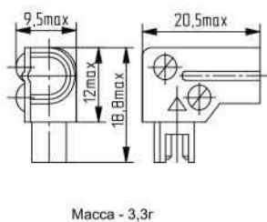
Рисунок 8 4-контактная вилка в металлическом или пластмассовом угловом кожухе РШ2Н-6, РШ2НМ-6
